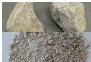
кварцит
